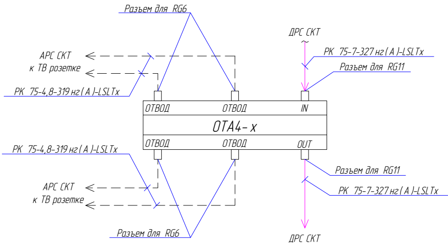
Схема подключения ответвителя ОТА 4- XX для 4- и абонентов
