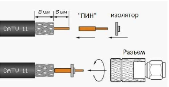
Инструкция по монтажу и сборке ВЧ разъема для кабеля типа RG11 (PK 75-7- xx)
