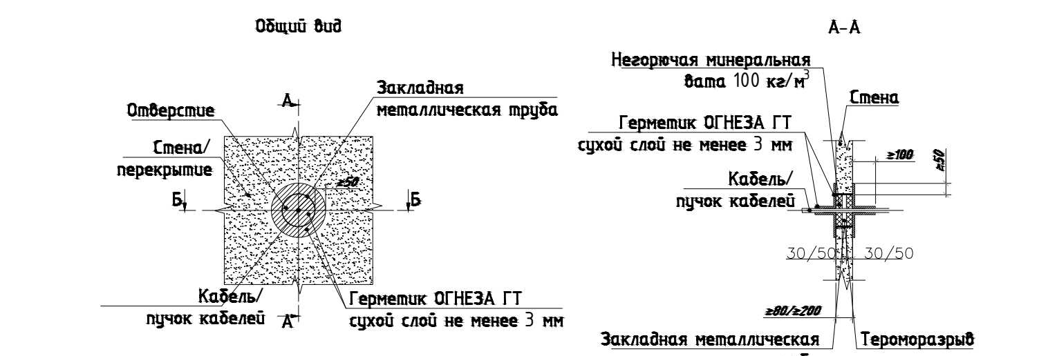
Типовой монтаж кабельной проходки в закладной трубе для стен и перекрытий с требуемым пределом огнестойкости с площадью от 300 м² (ЕИ1500/С200 мн (ЕИ1500))
