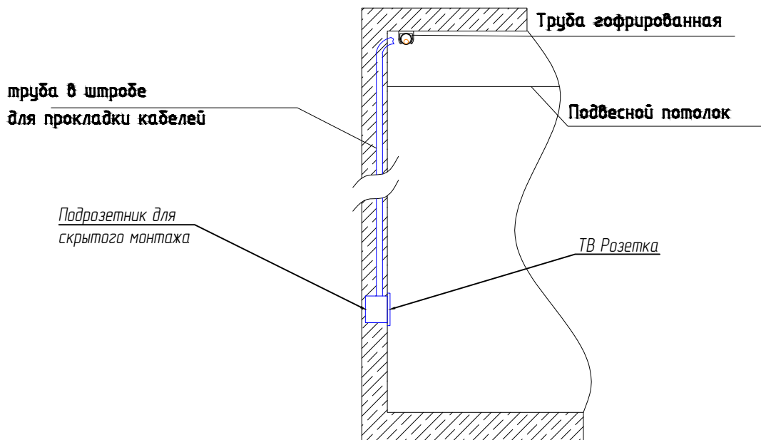
Разрез 1-1
