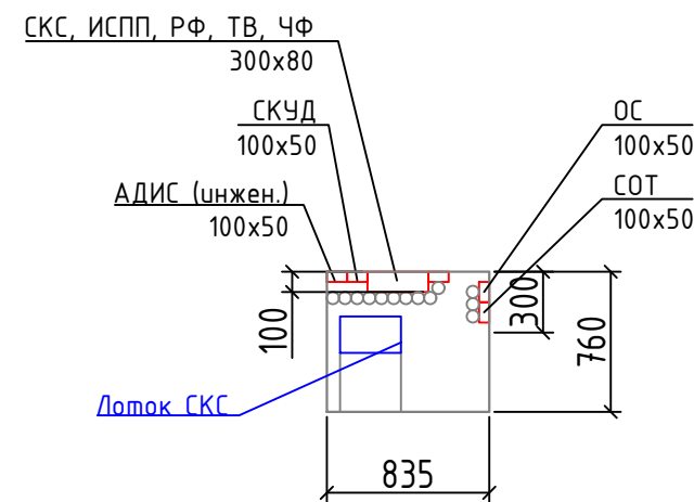
Вид В (вид сверху)
